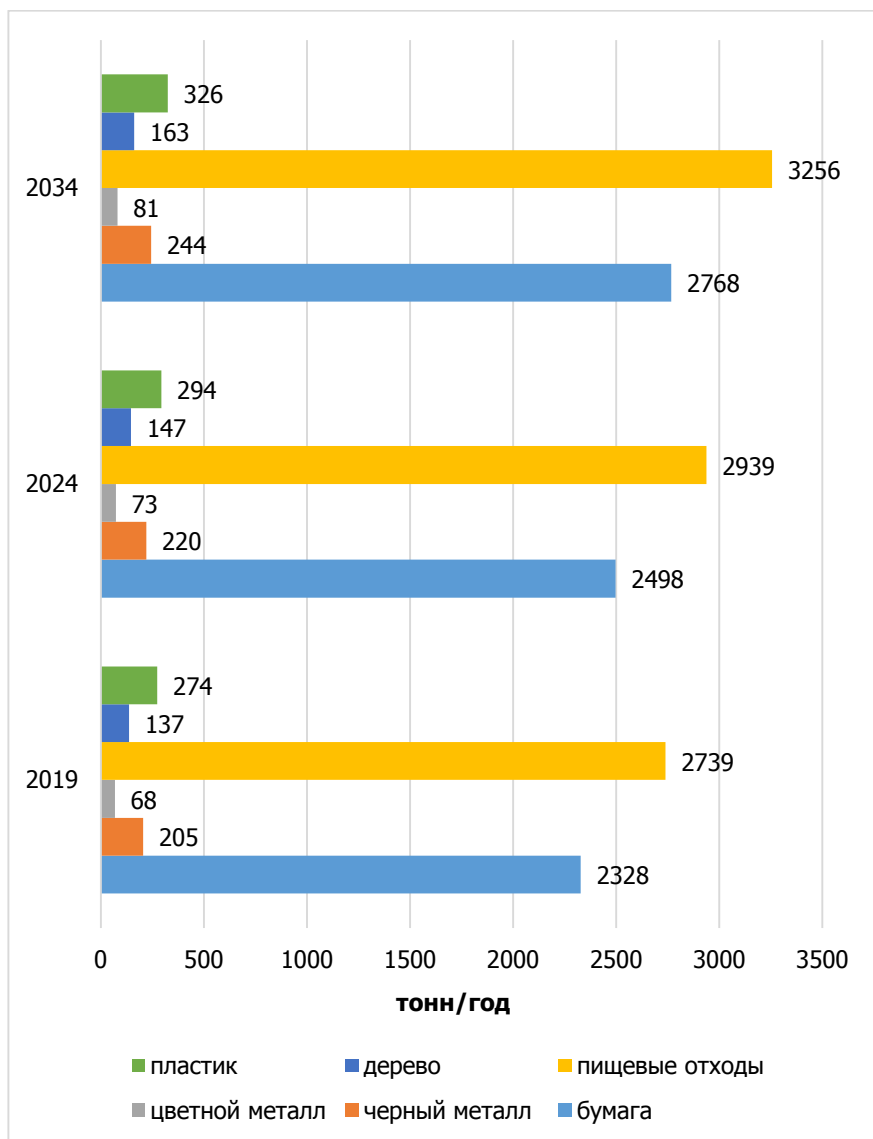
Рисунок 3.3 – Покомпонентный состав ТКО от населения в МО «Рощинское городское поселение» (в тоннах по годам)
