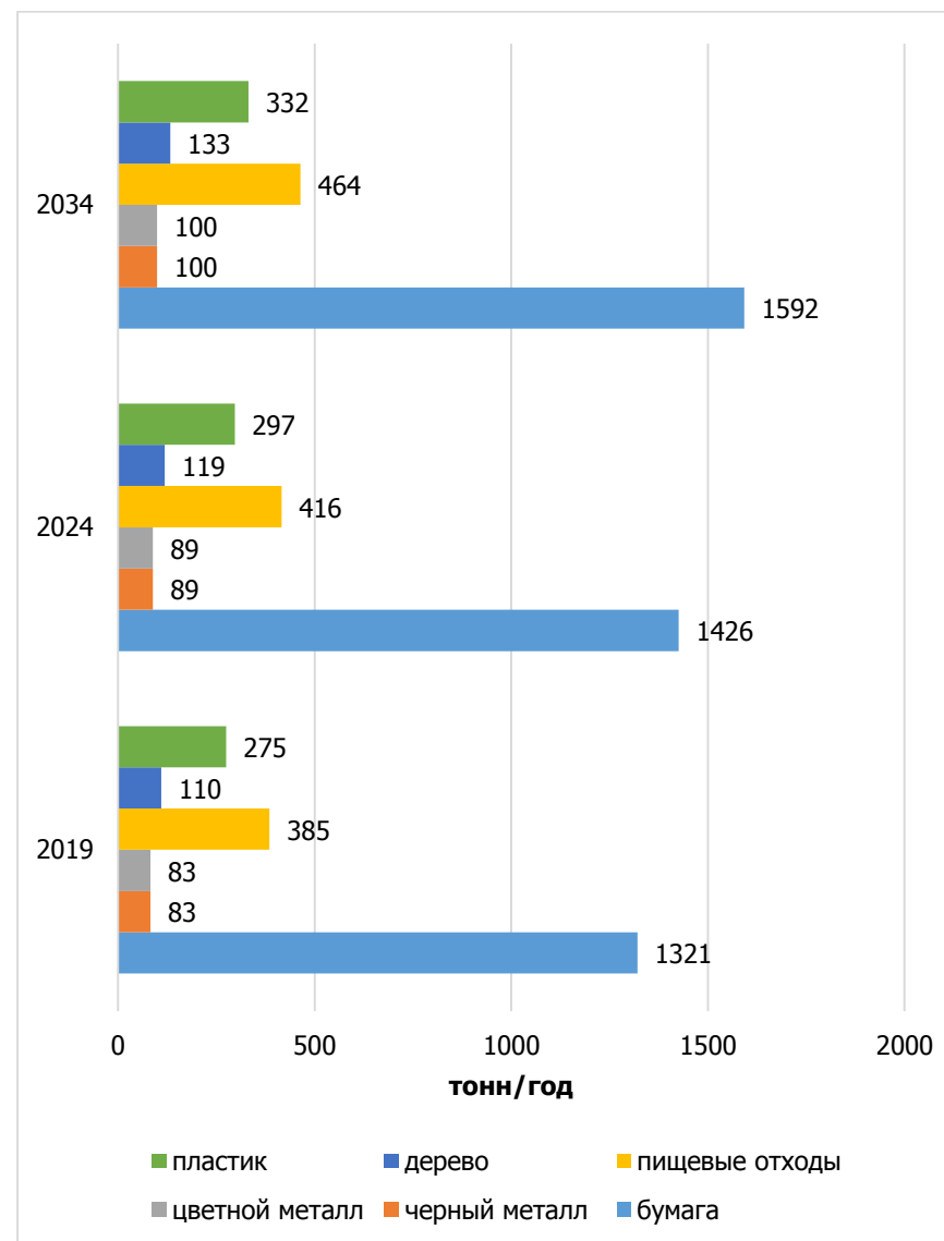
Рисунок 3.4 – Покомпонентный состав ТКО от организаций и предприятий в МО «Рощинское городское поселение» (в тоннах по годам)
